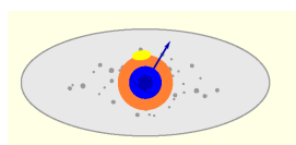
Obr. 2g. Tvorba silikátového obalu.
