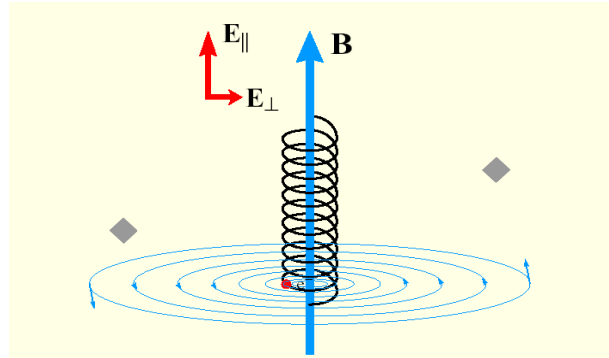
Obr. 2b.: Fyzikálny princíp impulzného mg. poľa. Elektrón pohybujúci sa pozdĺž mg. siločiar ( \mathbf{B} ) rotačným pohybom vytvára lineárny el. prúd ( \mathbf{E}_{||} ). Ten generuje kruhové mg. pole, ktoré magnetizuje feromagnetické planetesimály.
