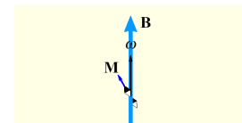
Obr. 2e. Zachovanie mg. momentu po doznení výboja a získanie rotácie spojených častíc ako dôsledok zachovania ich momentov hybnosti.
