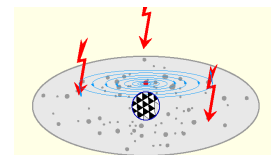
Obr. 2f. Zväčšovanie jadra viacnásobnými výbojmi
