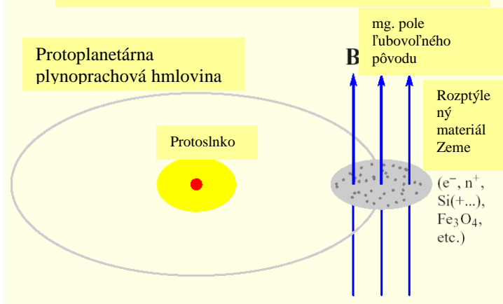
Obr. 2a.: Model tvorby Zeme akreciou. V plynoprachovej počiatkovej hmlovine sa tvorí z rozptýleného materiálu zárodok Zeme. Prítomné je aj magnetické pole rôzneho pôvodu.
